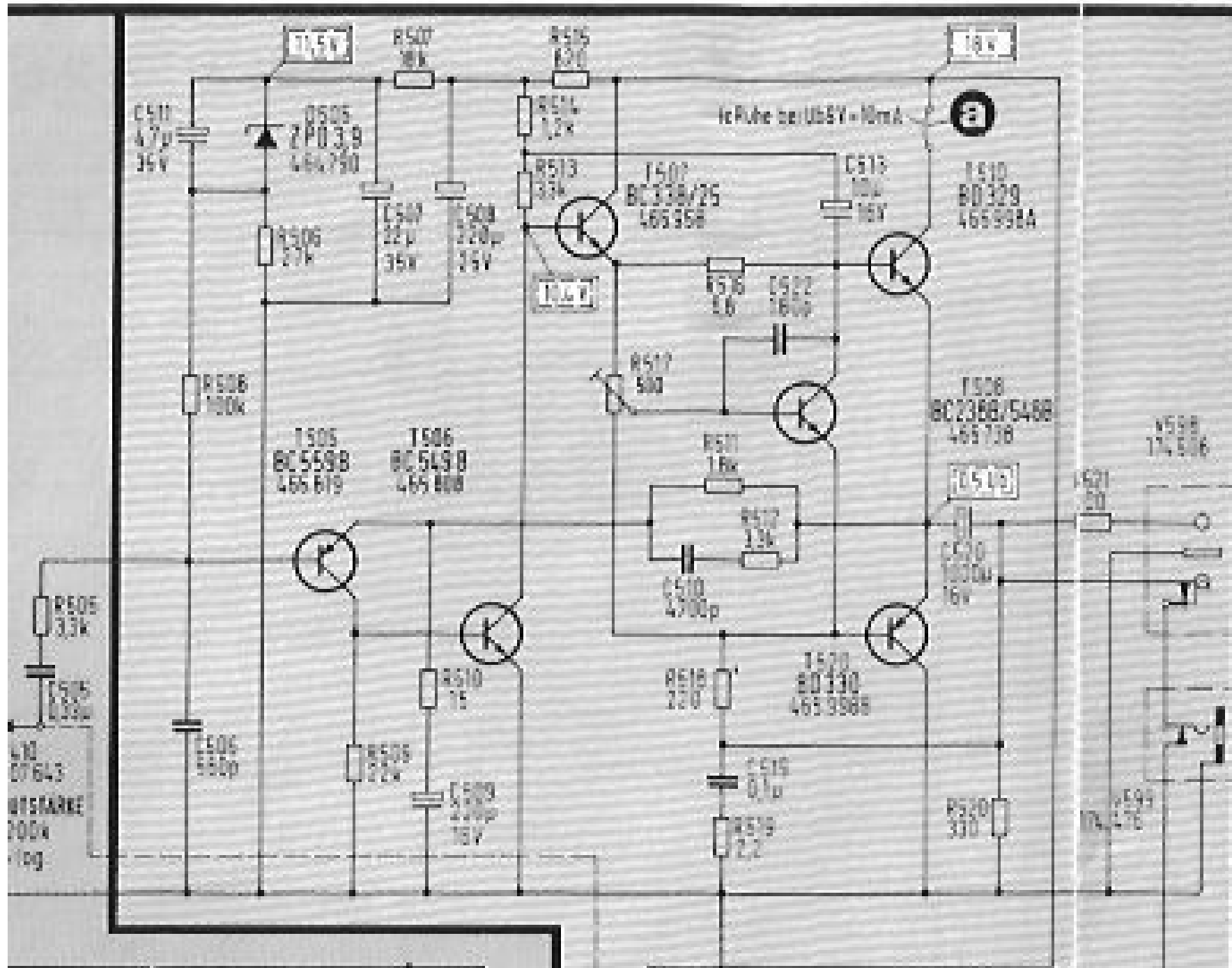
NordMende Globetrotter 808 output stage.
